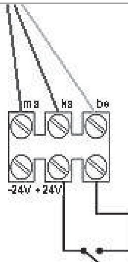
Рисунок 8.3 С КОМНАТНЫМ ТЕРМОСТАТОМ
