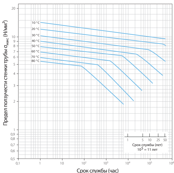
Срок службы труб Uponor HDPE (Uponor Supra)
