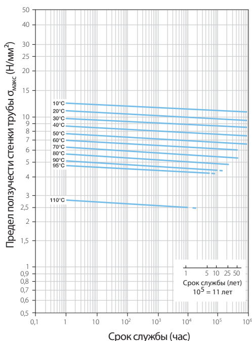
Срок службы труб Uponor PE-Xa
