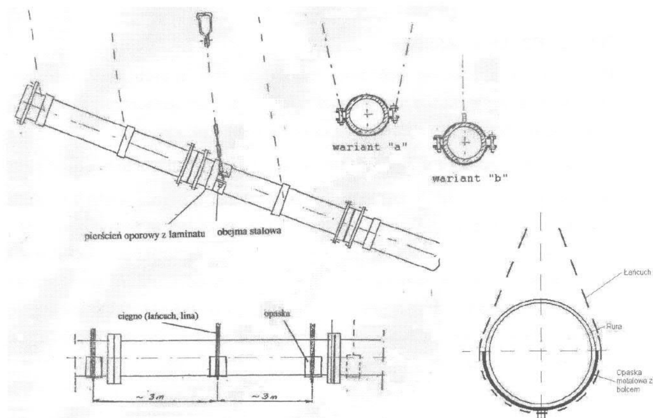
Przykłady mocowania rur na zawiesiach.
