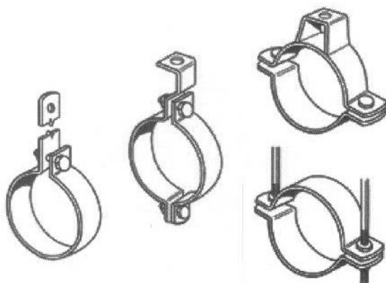
Sztywne zawiesia
