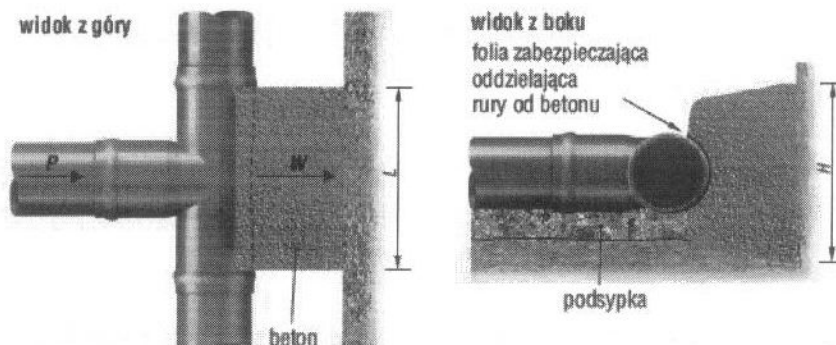
Blok oporowy dla trójnika
