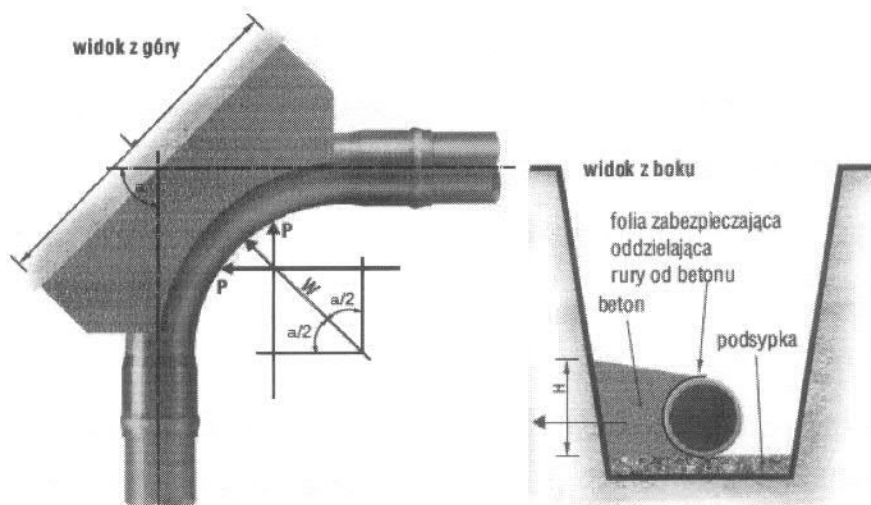
Blok oporowy kolana lub łuku
