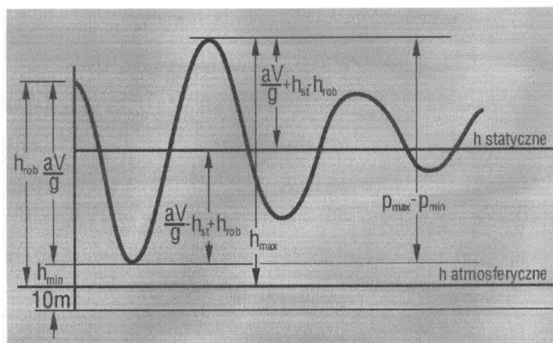
Przebieg fali uderzenia hydraulicznego
