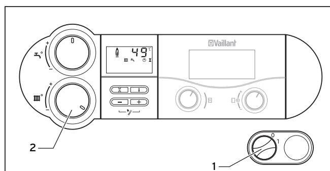
Мал. 4.7 Настроювання температури лінії подачі з використанням регулювального пристрою
