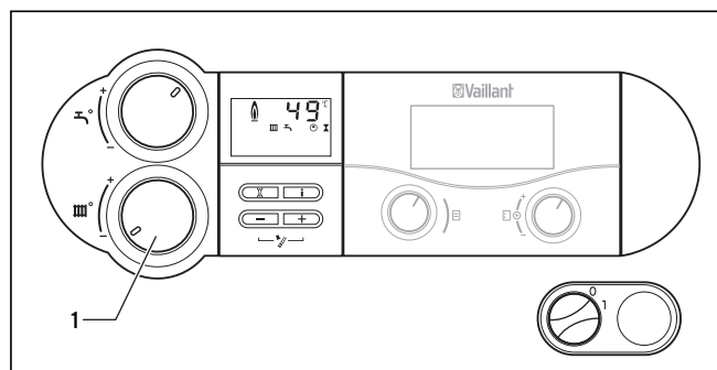
Рис. 4.9 Отключение режима отопления (летний режим)
